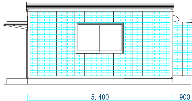
B面 立面図 S=1/50
