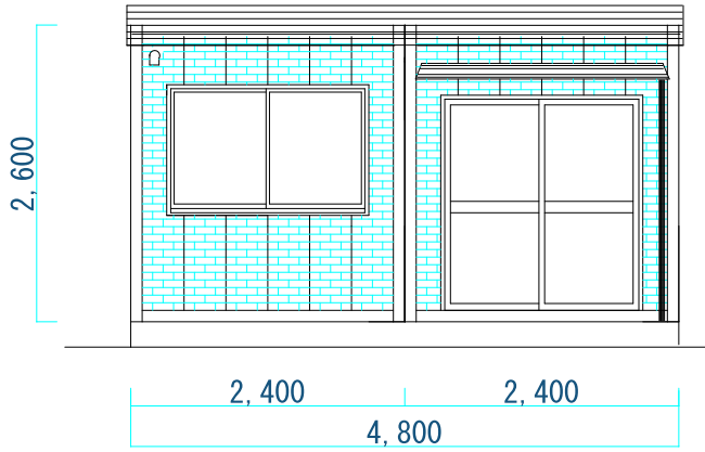
C面 立面図 S=1/50
