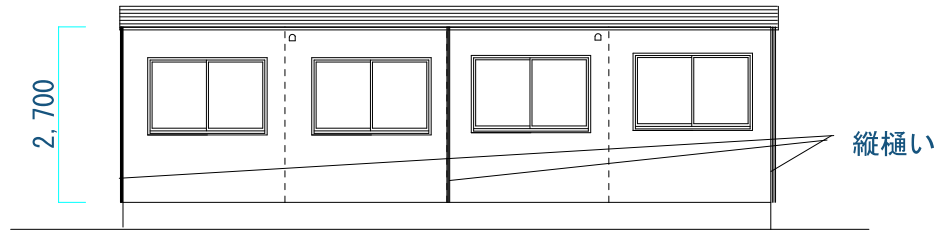
A面立面図 S=1/75
