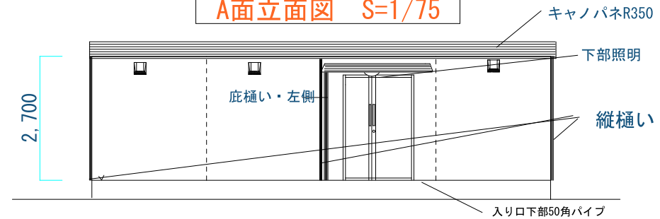
C面立面図 S=1/75
